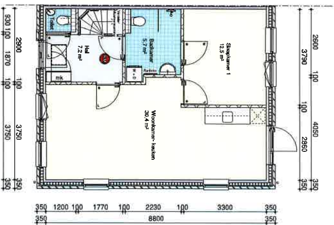
Begane grond
