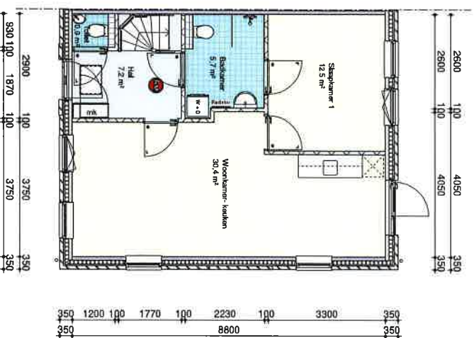
Begane grond
