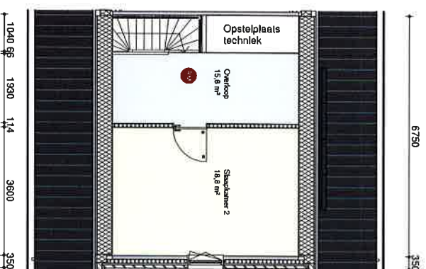
1e Verdieping
