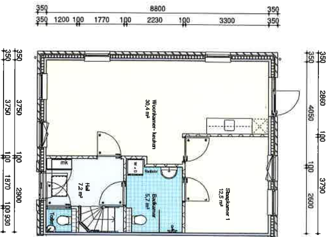
Begane grond
