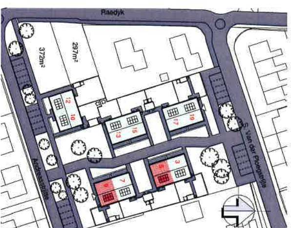
Situatie
