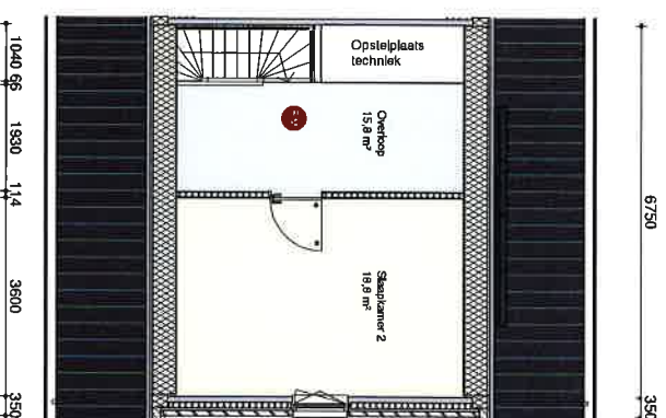
1e Verdieping
