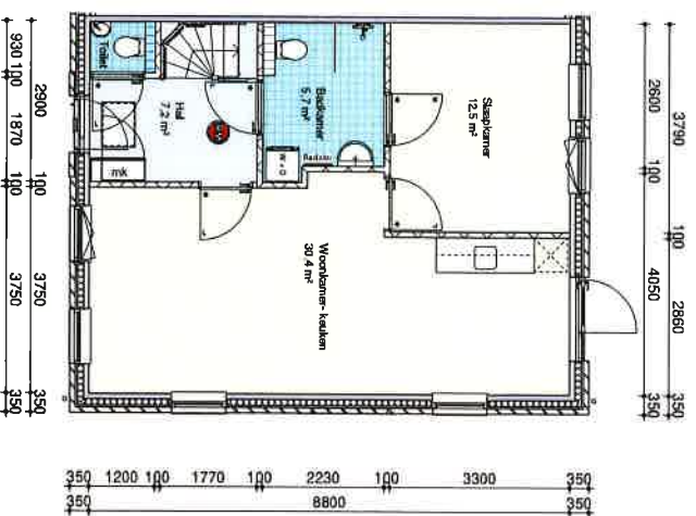
Begane grond
